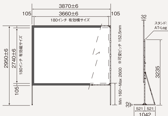
■ 180インチ組立式スクリーン(シングルフレーム)
