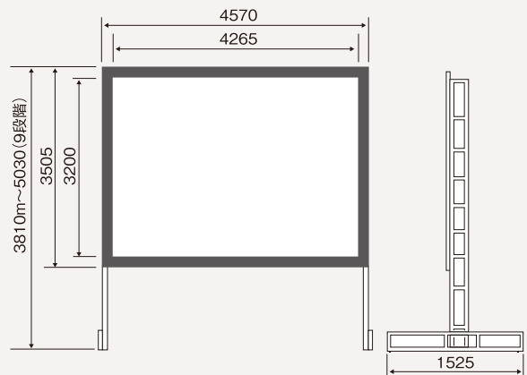
■ 210インチ組立式スクリーン(トラスフレーム)
