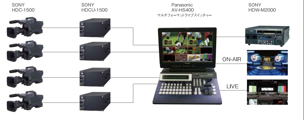
《HDカメラ4カメ中継システムの一例》
